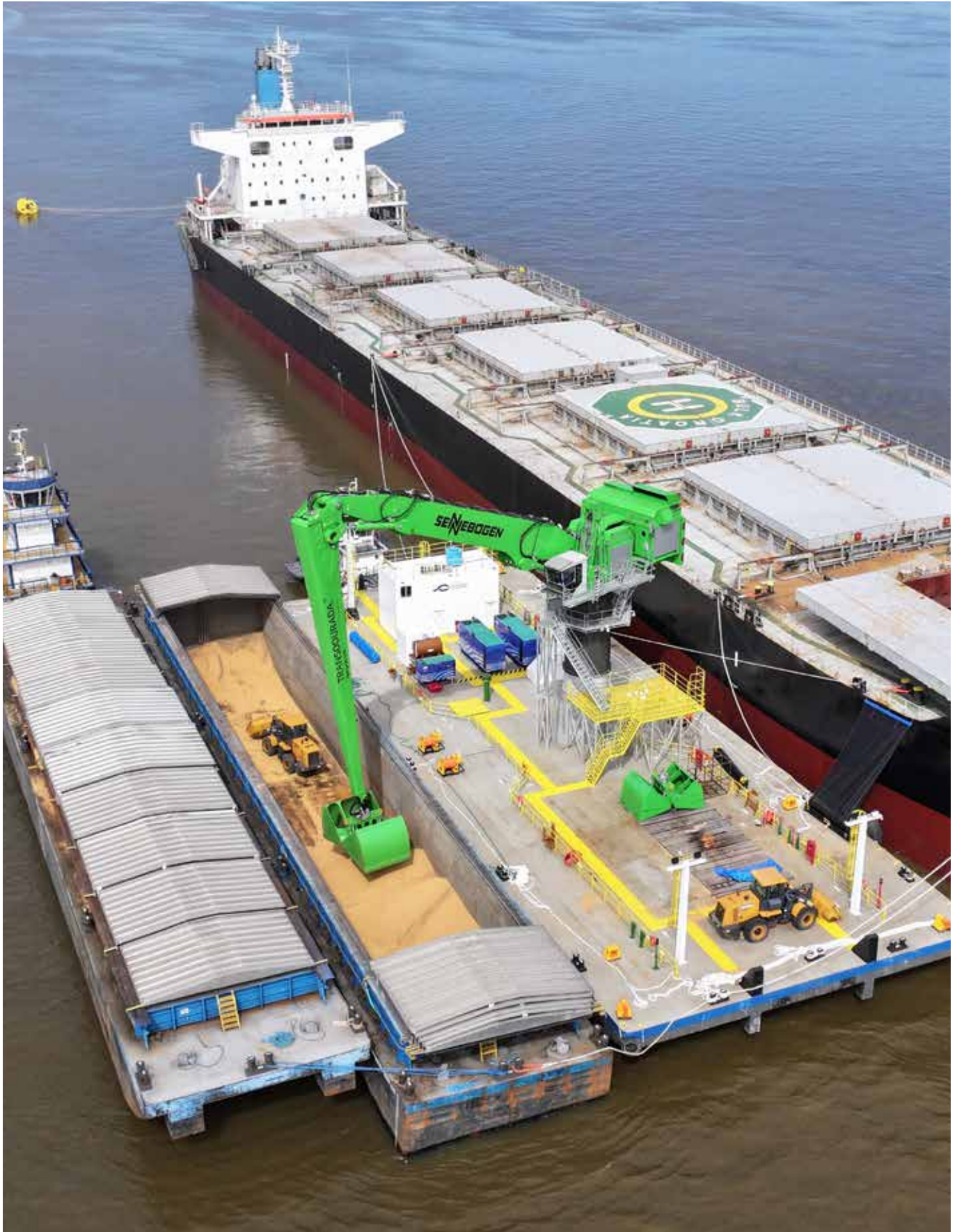
Schiff-zu-Schiff-Transfer; Brasilien
