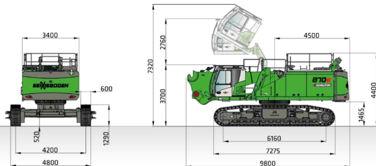
870 DEMOLITION GRUNDMASCHINE INKL. OBERWAGEN-GELÄNDER UND GEGENGEWICHT, TRANSPORTGEWICHT CA. 92 t INKL. GEGENGEWICHT CA. 26 t
