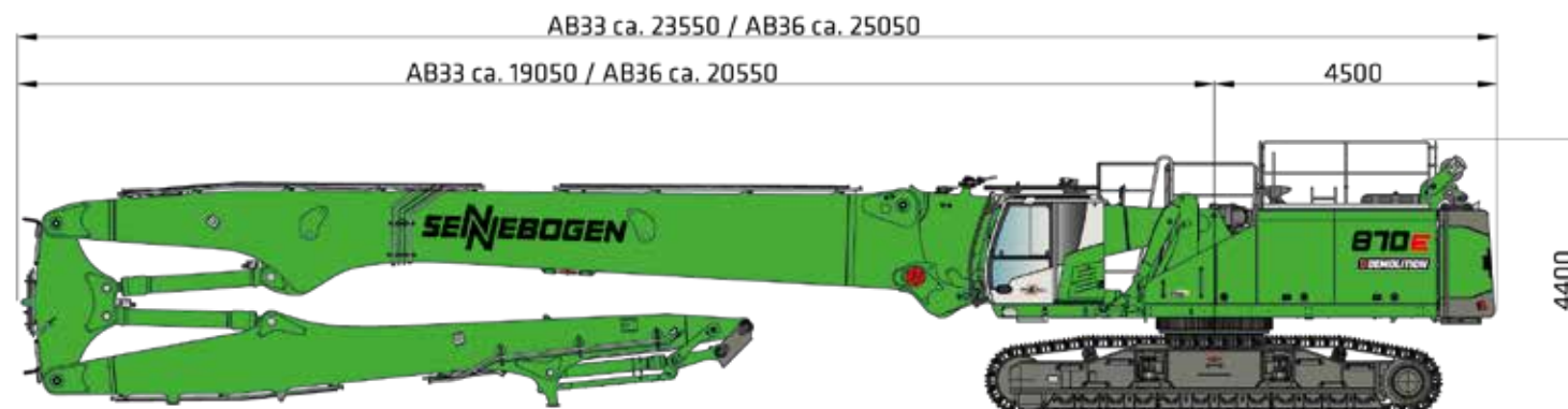
870 DEMOLITION MIT UNTERWAGEN T102/420 UND 3-TEILIGEM ABRUCH-AUSLEGER, HYDRAULISCH HOCHFABRBARER KABINE MAXCAB, 30° NEIGBAR, ULM EINSATZGEWICHT CA. 114 t - 117 t (OHNE WERKZEUG)
