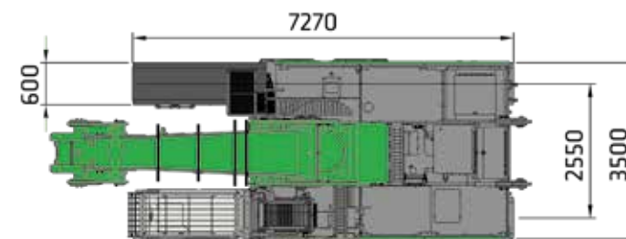
870 DEMOLITION GRUNDMASCHINE UNTERWAGEN EINTELESKOPIERT OHNE GEGENGEWICHT
