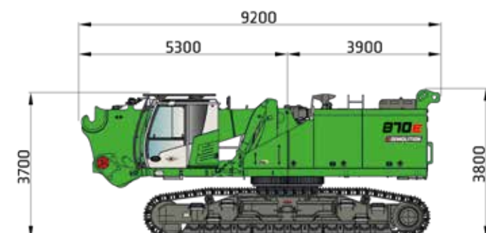
* = Transportbreite
