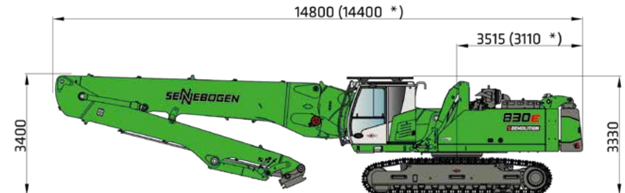
830 DEMOLITION VARIO TOOL, AB17 MIT UNTERWAGEN T41/380, ABBRUCHAUSTRÜSTUNG AB17, HYDRAULISCH HOCHFÄHRBARE KABINE MAXCAB, 30° NEIGBAR, HYDRAULISCHER BALLASTABLAGE (OPTION), EINSATZGEWICHT: 51 t
