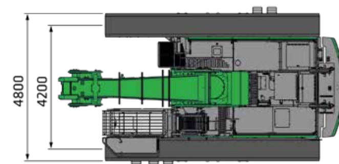
870 DEMOLITION GRUNDMASCHINE UNTERWAGEN AUSTELESKOPIERT INKL. GEGENGEWICHT
